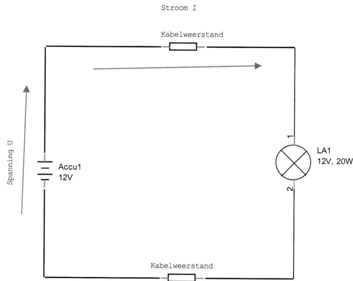
Figuur 2: Stroomkring met realistische bedrading
